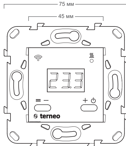
Рисунок 1. Габаритные размеры
